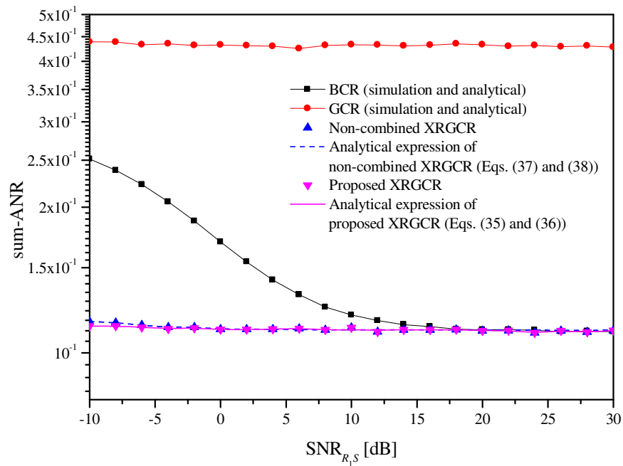
Fig. 9. Sum-ANR versus SNR_{R_1S} .
